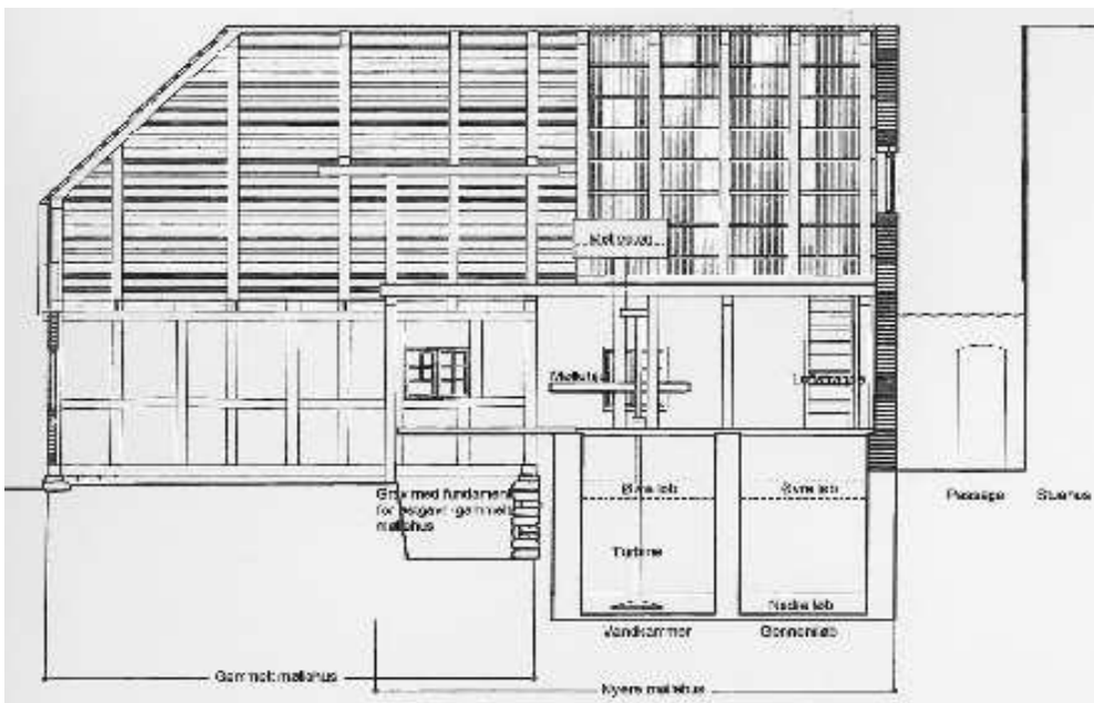
Snit gennem møllehuset, med vandturbinen vist i venstre gennemløb.
